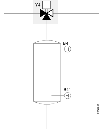
Isı kaynağı kapatma vanası aküm.tankı
