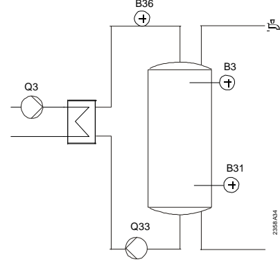
Harici ısı eşanjörlü ve besleme pompalı, ara resirkülasyon pompalı DHW tankı
