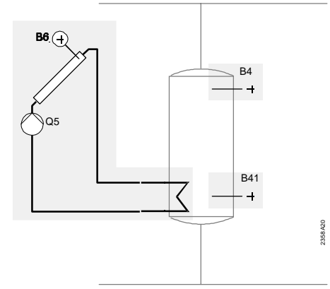
Akümülayon tankı besleme
