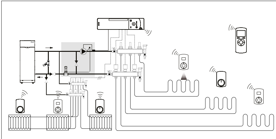
Isı pompası ile kombine döşemeden ısıtma sistemi
