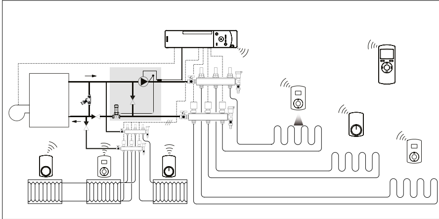
Kazan ile kombine döşemeden ısıtma sistemi
